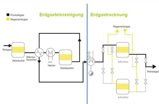
Anlagenschema
