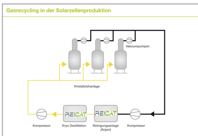
Anlagenschema
